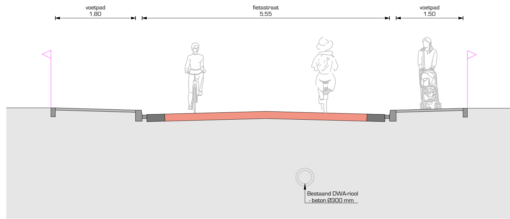
Principeprofiel: B-B Schaal: 1:50
